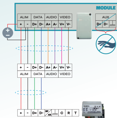
INTERPHONE VIDÉO 4 À 20 BOUTONS SAILLIE
