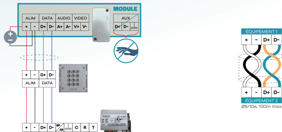
CLAVIER CODÉ AVEC LECTEUR DE BADGES MAINS-LIBRES « SLIM »
